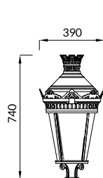
CHENONCEAUX II Post top
